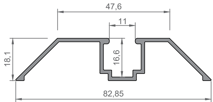
16004 GUÍA INFERIOR
