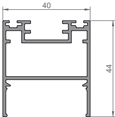
16006 HOJA CORREDERA
