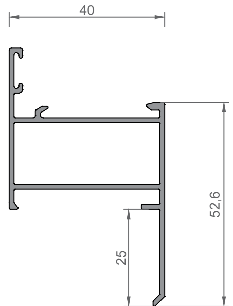
11021 Marco solape
