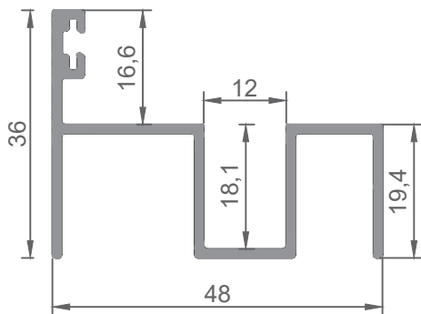
4653 MARCO - GUÍA INFERIOR
