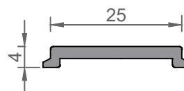
11009 Pletina falleba 40x20
