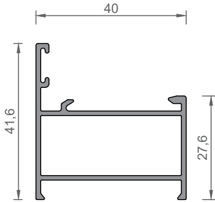
11001 Marco ventana
