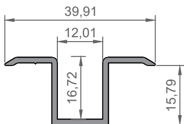
16006 GUÍA INFERIOR EMBUTIDO
