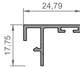
16010 PERFIL INVERSOR
