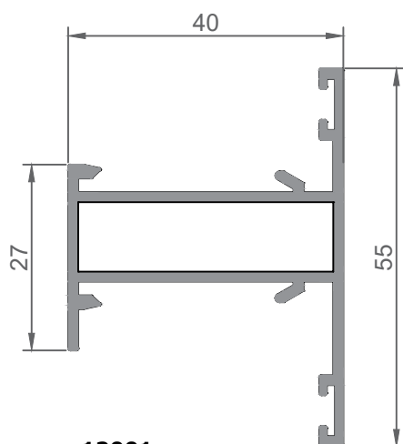
12001 Invesor mallorq.
