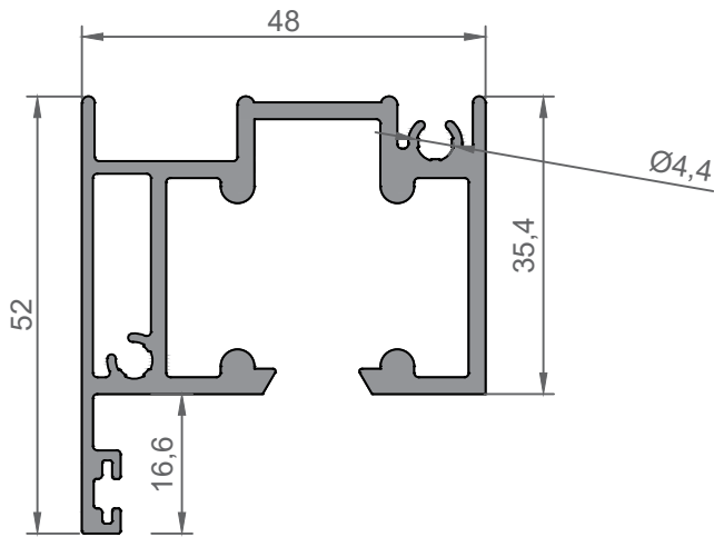
4652 GUÍA SUPERIOR
