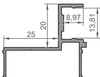
19297 Suplemento LISTONES
