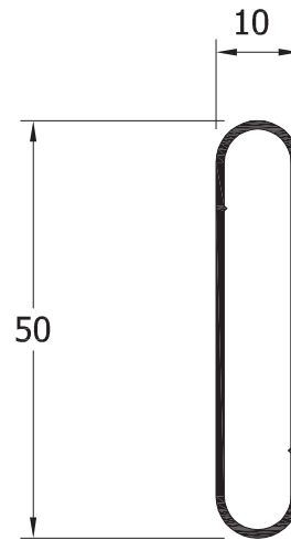
12003 Lama fija mallorq.
