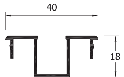
12004 Acople terminal mallorq.
