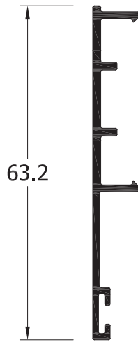
16005 Tapa guia superior forjado
