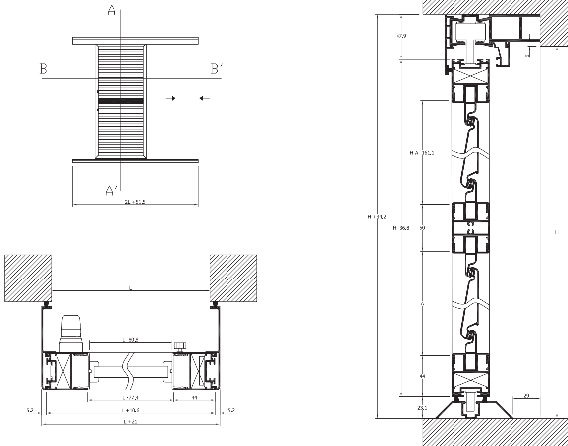
Guia entre forjados
