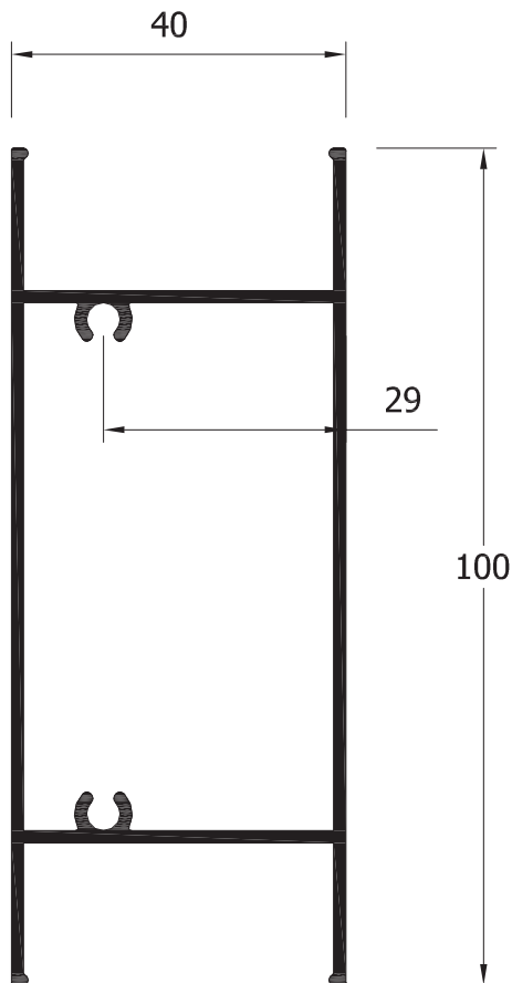
12010 Divisor zócalo grande mallorq.
