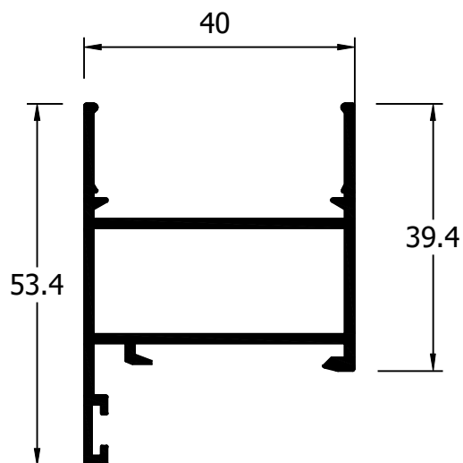
12000 Hoja ventana mallorq.
