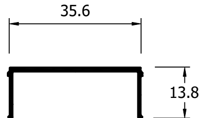
041 0 Tapa U mallorquina
