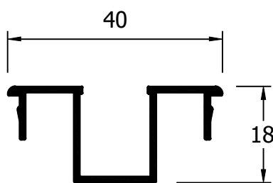
12004 Acople terminal mallorq.
