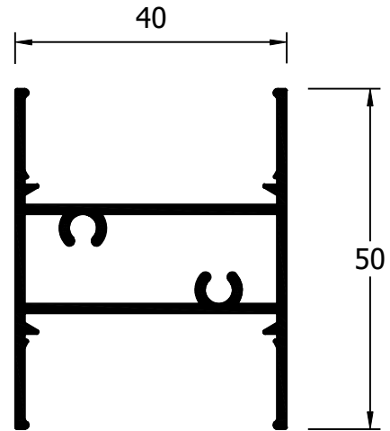
12007 Divisor peq. mallorq.
