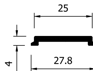
11009 Pletina falleba 40x20
