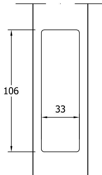
Mecanizado Tapa Plana (18003)
