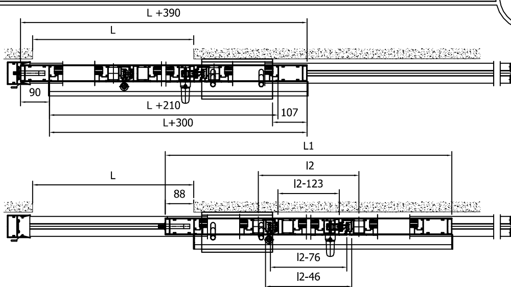
Medidas de corte CORREDERA - 1 hoja con Puerta abatible ( mm )
