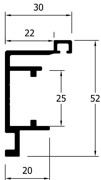
18005 Acople Batiente Pilastra
