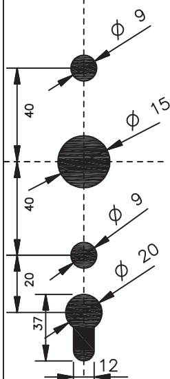
CREMONA
