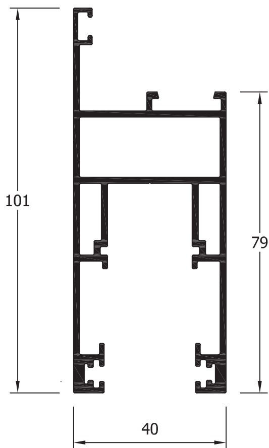
25011 Hoja 250 Kg.
