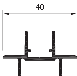
25010 Unión 4 hojas
