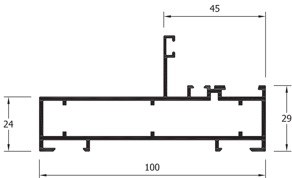
25007 Marco fijo
