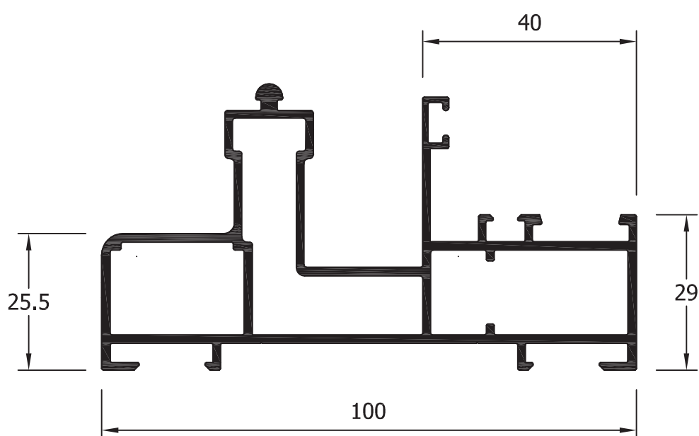
25014 Marco monocarril
