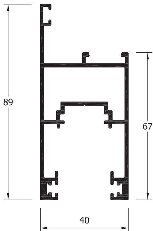
25008 Hoja 150 Kg.
