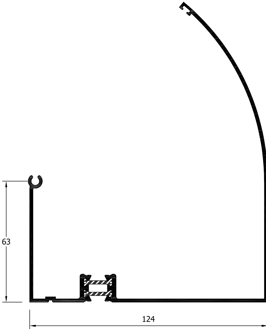
ALF-52 Esquinero Compacto RPT Macho 120 mm
