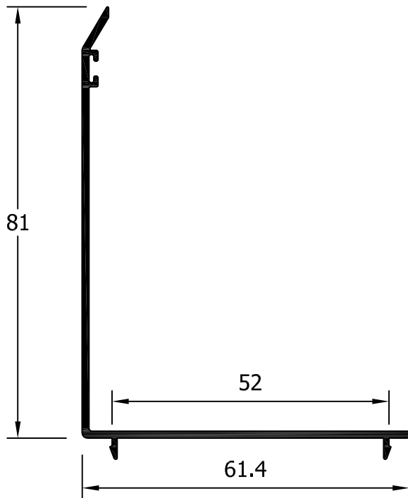
02-041C Tapajuntas Clip 81 mm
