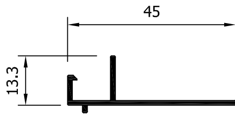
22044 Acople Registro 40 mm EU-75
