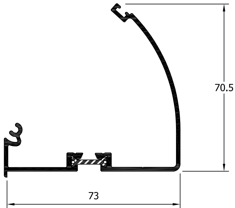
14010 Esquinero graduable hembra 70 RPT
