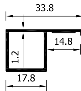
7147 Premarco PLADUR 34 mm
