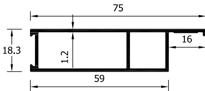
7148 Premarco PLADUR 75mm
