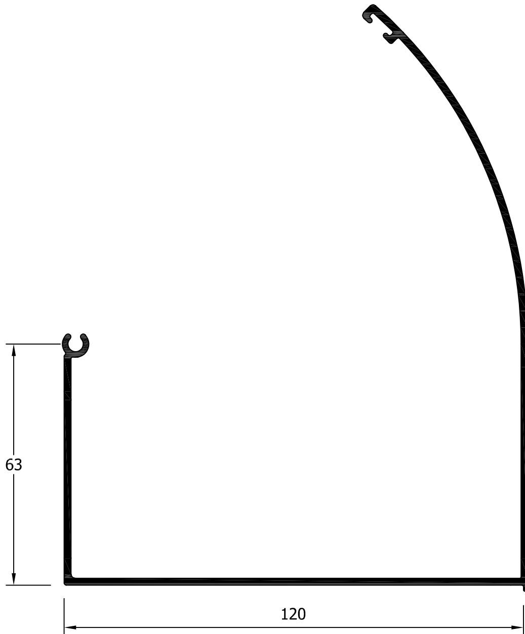
31014 Esquinero Graduable Macho Compacto 120 mm
