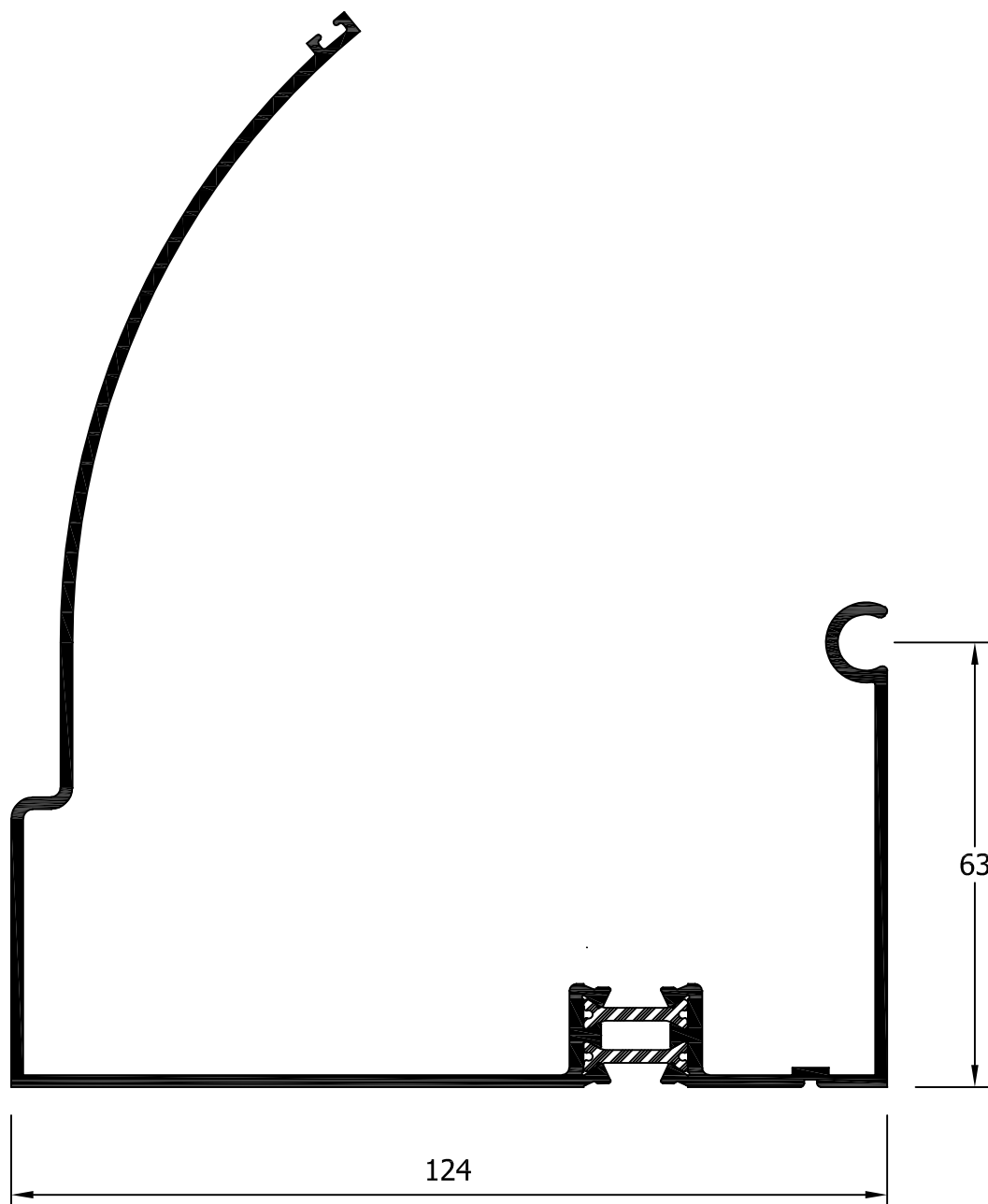
ALF-51 Esquinero Compacto RPT Hembra 120 mm
