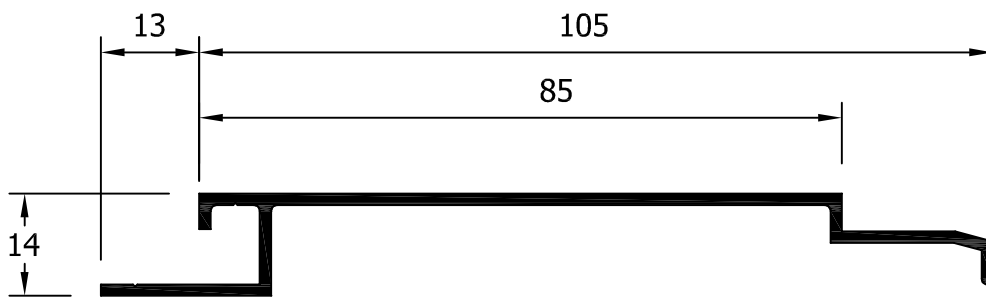
14312 ( 9 lamas por metro )
