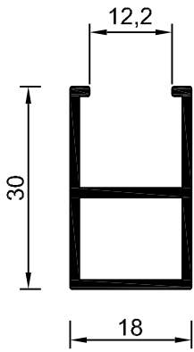
REF-14002 PERFIL U. 30X18
