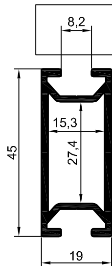
REF-18923 Perfil tec.divisor 45x19
