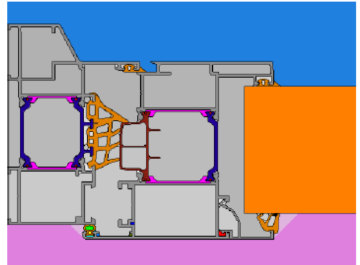
Uf Marco: 2.2 W/m2K
