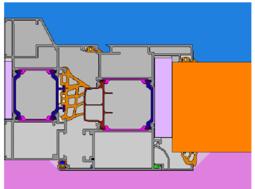
Uf Marco: 1.9 W/m2K
