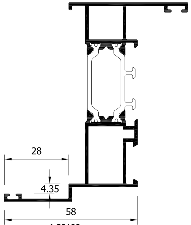
* 80190 Marco tapajuntas resalte.28 mm
