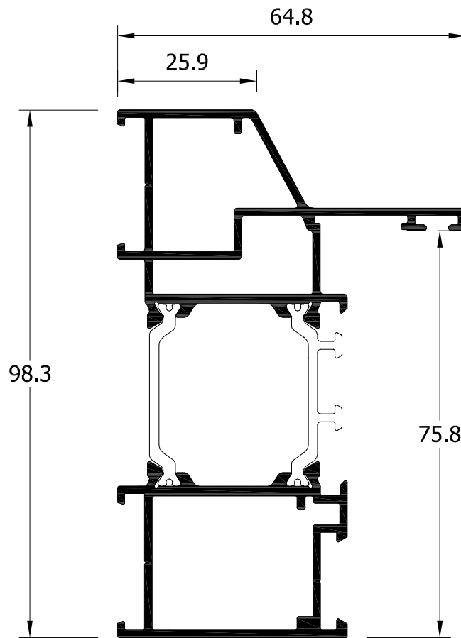
80191 Marco puerta escarparte
