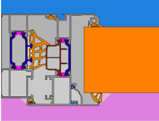
Uf Marco: 2.2 W/m2K
