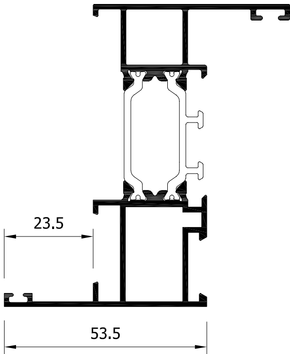
80187 Marco tapajuntas 23 mm
