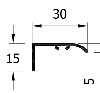
23011 Tapajuntas 30 s/clip
