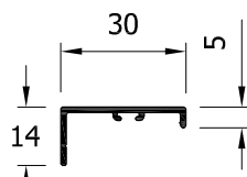
75161 Tapajuntas recto 30 s/clip
