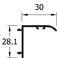
24007 Solape clipado 30 mm
