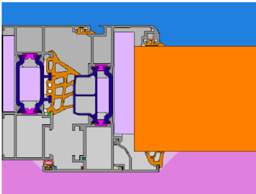
Uf Marco: 1.6 W/m2K
