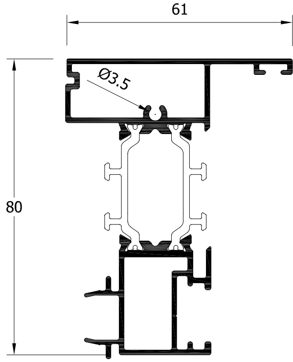
80188 Inversor
