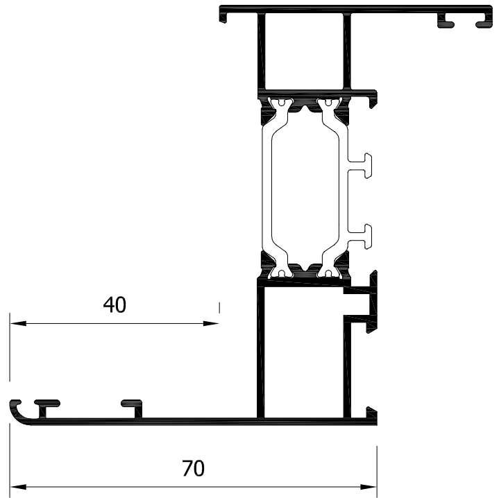
* 80189 Marco tapajuntas 40 mm
