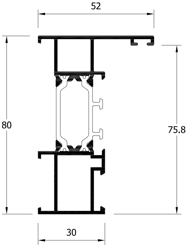
80181 Marco ventana
