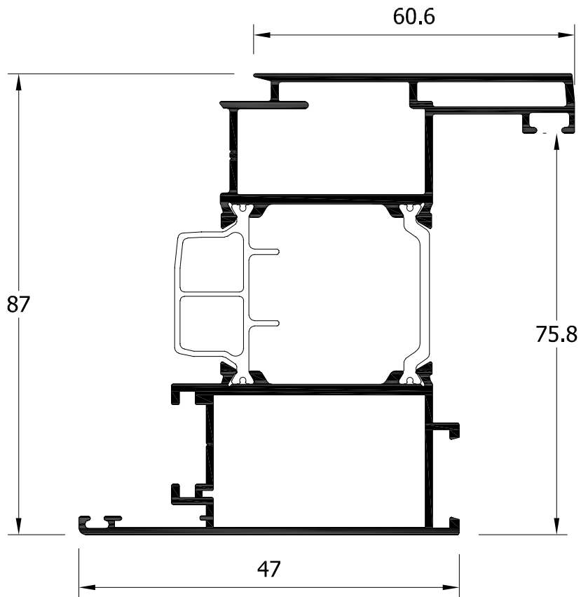
80193 Hoja puerta recta
