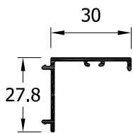
75160 Solape recto clipado 30 mm
