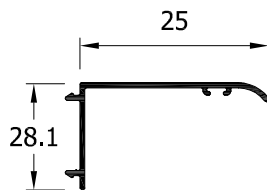
24008 Solape clipado 50 mm
