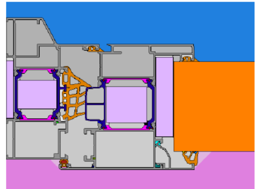
Uf Marco: 1.4 W/m2K
